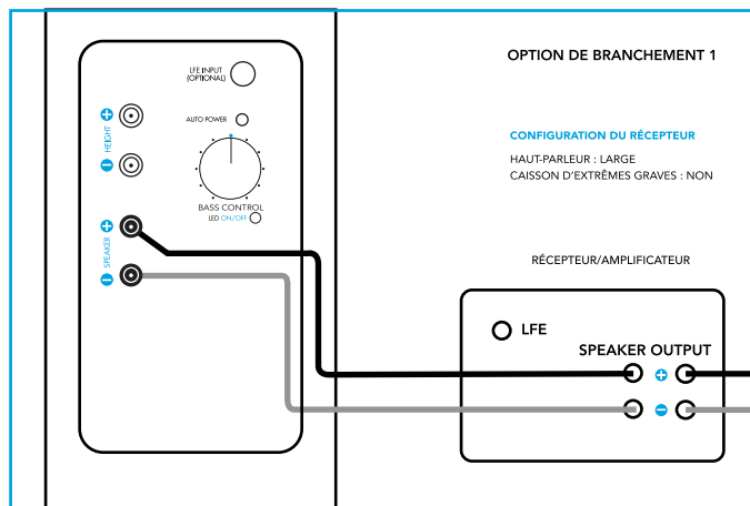
FIGURE 4 – Schéma du branchement niveau du haut-parleur seulement
