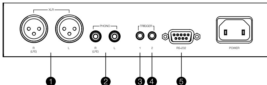
3. ábra A DB mélysugárhó csatlakozó aljzatai
